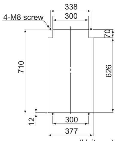
FR-A7CN14
