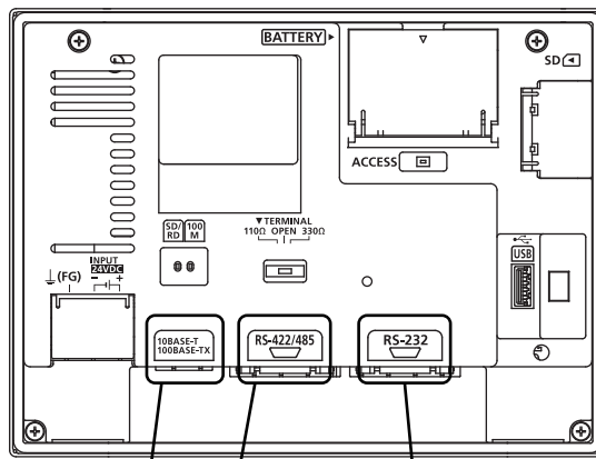
Standard I/F-2(RS-232) Standard I/F-1(RS-422/485) Standard I/F-4(Ethernet)
